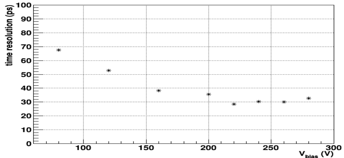
USTC-IME_W24-P41_1x2-LGAD-far_8e14
