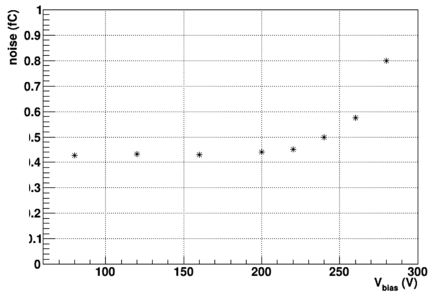
USTC-IME_W24-P41_1x2-LGAD-far_8e14
