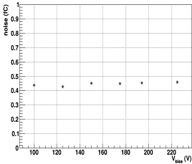
IHEP-IME_V1R2-32-1x2-LGAD2_8e14
