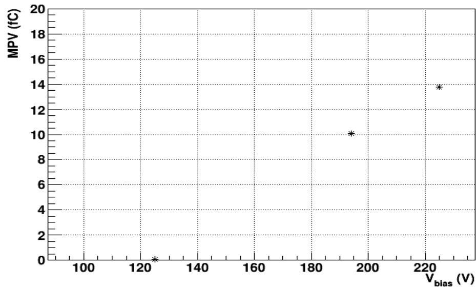
IHEP-IME_V1R2-32-1x2-LGAD2_8e14
