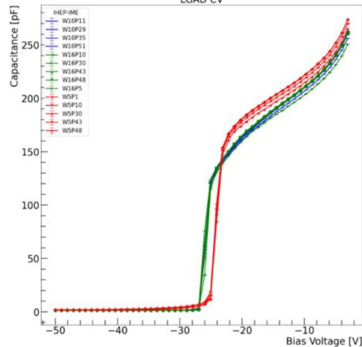
LGAD CV
