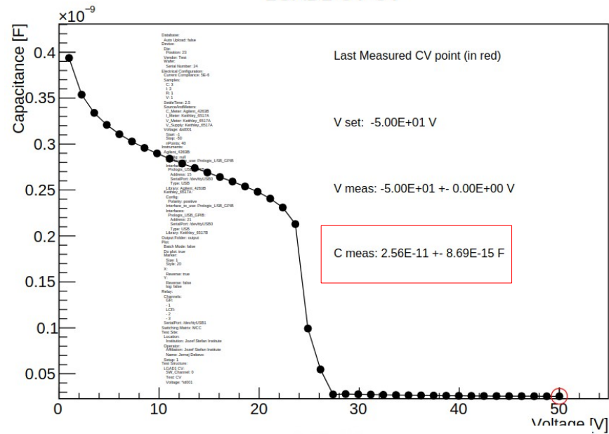
LGAD CV
