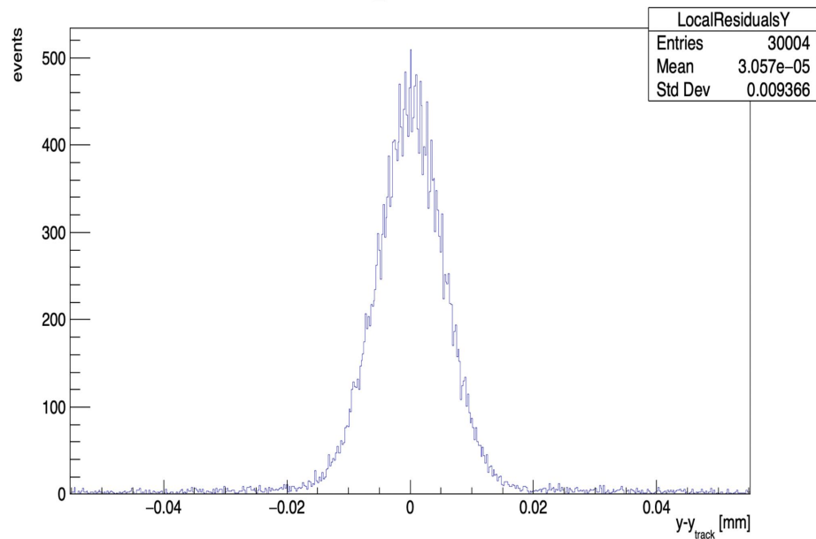
MIMOSA26_3Local Residual Y
