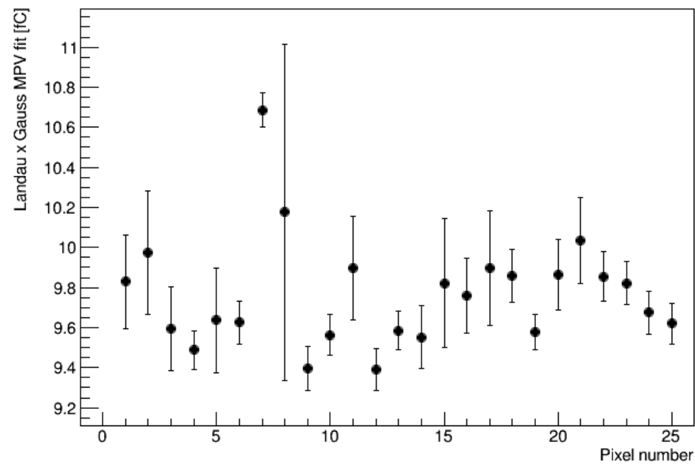
MPV per pixel
